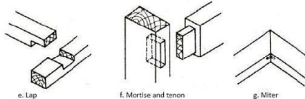
e. Lap
