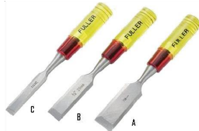
A - fiemer Chisel / B - Bevel Chisel / C - Mortise Chisel
