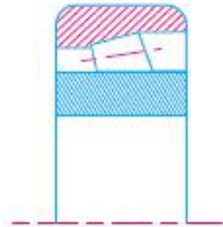
(d) Tapered roller.
